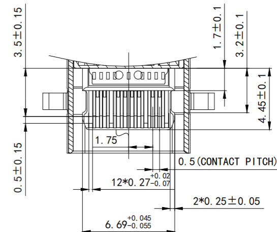
剖面 B-B
